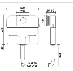
PARI - E.W.C. / E.W.C. CONCEALED
